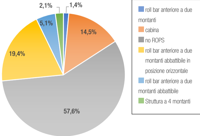
Fig. 8 – Ribaltamenti fatali verificatisi in Italia nel periodo 2008-2019 classificati in base al tipo di struttura protettiva installata (Rops)
